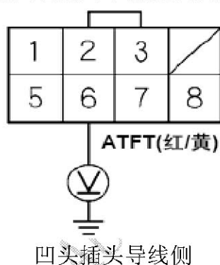
换档电磁阀导线线束插头
