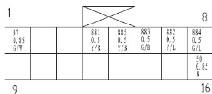
接ECU
