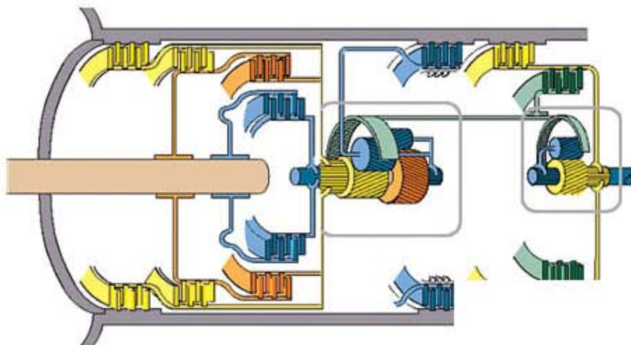
图 2 压力调节阀、减压阀位置图
