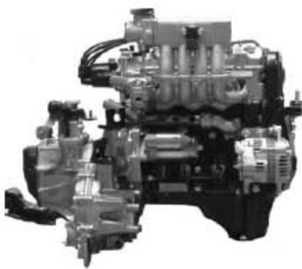
汽油机右视外形图:
