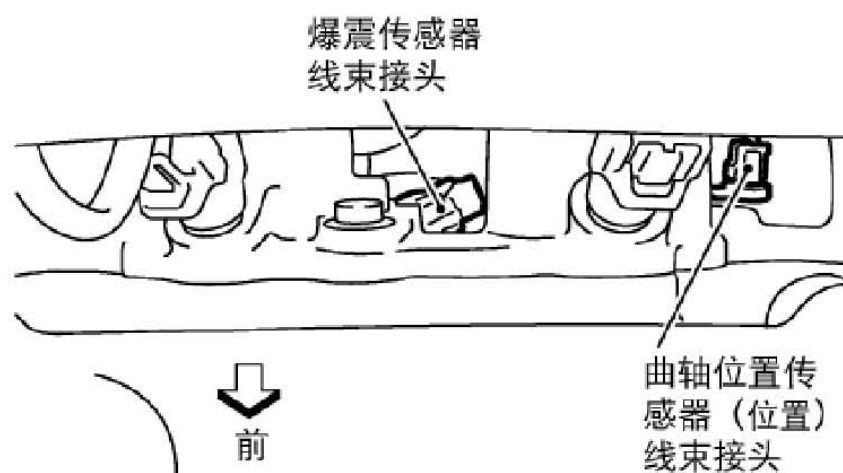
拆下发动机后的视图
