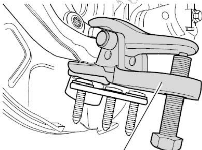
万向节拔出器
