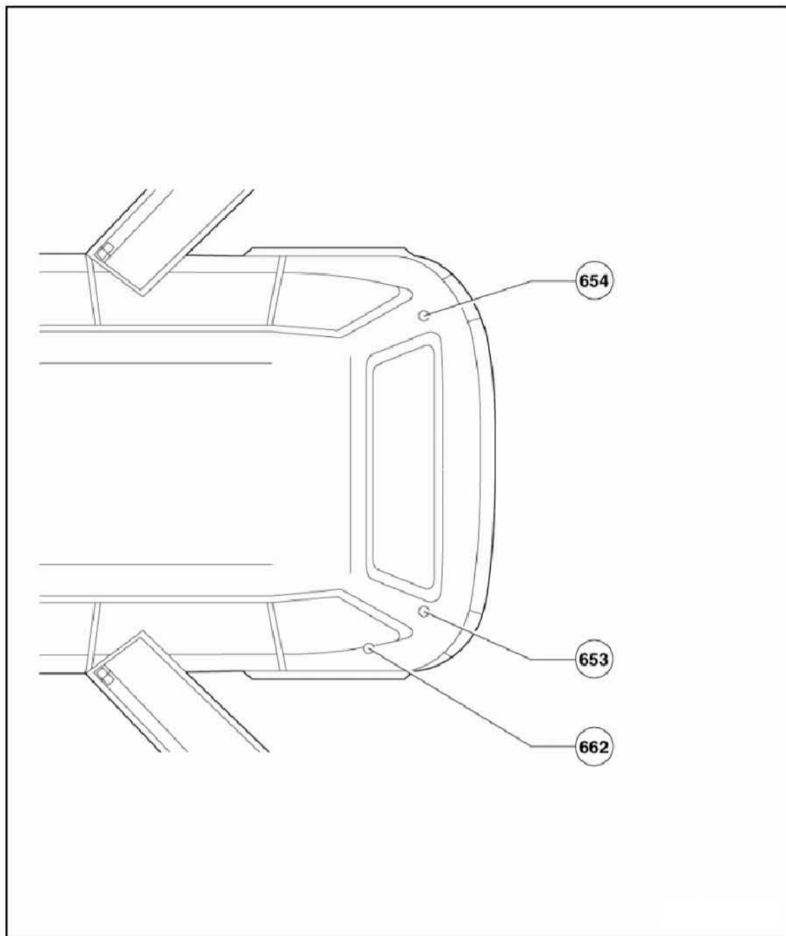
行李箱内所有接地点一览
