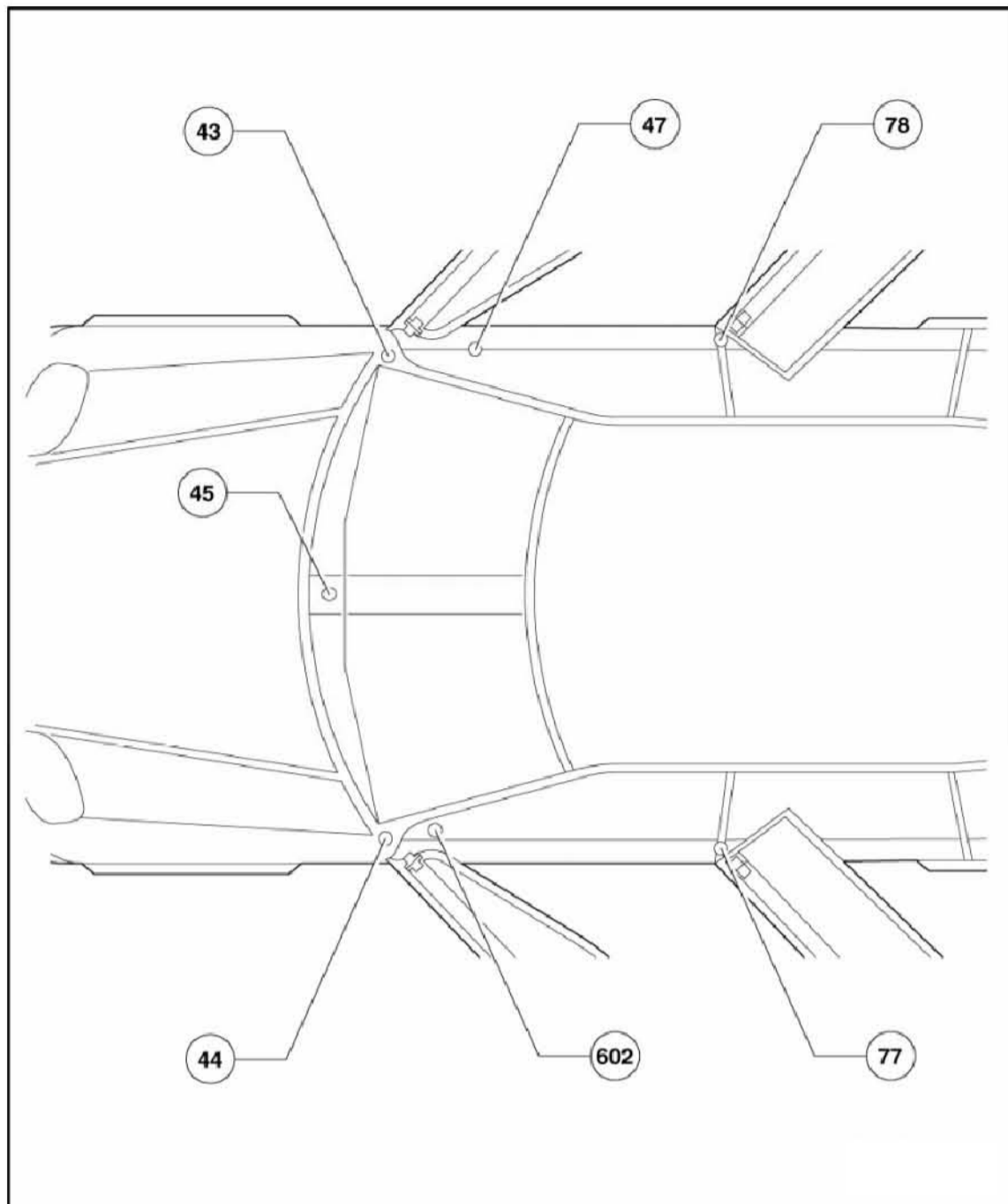
车内所有接地点一览
