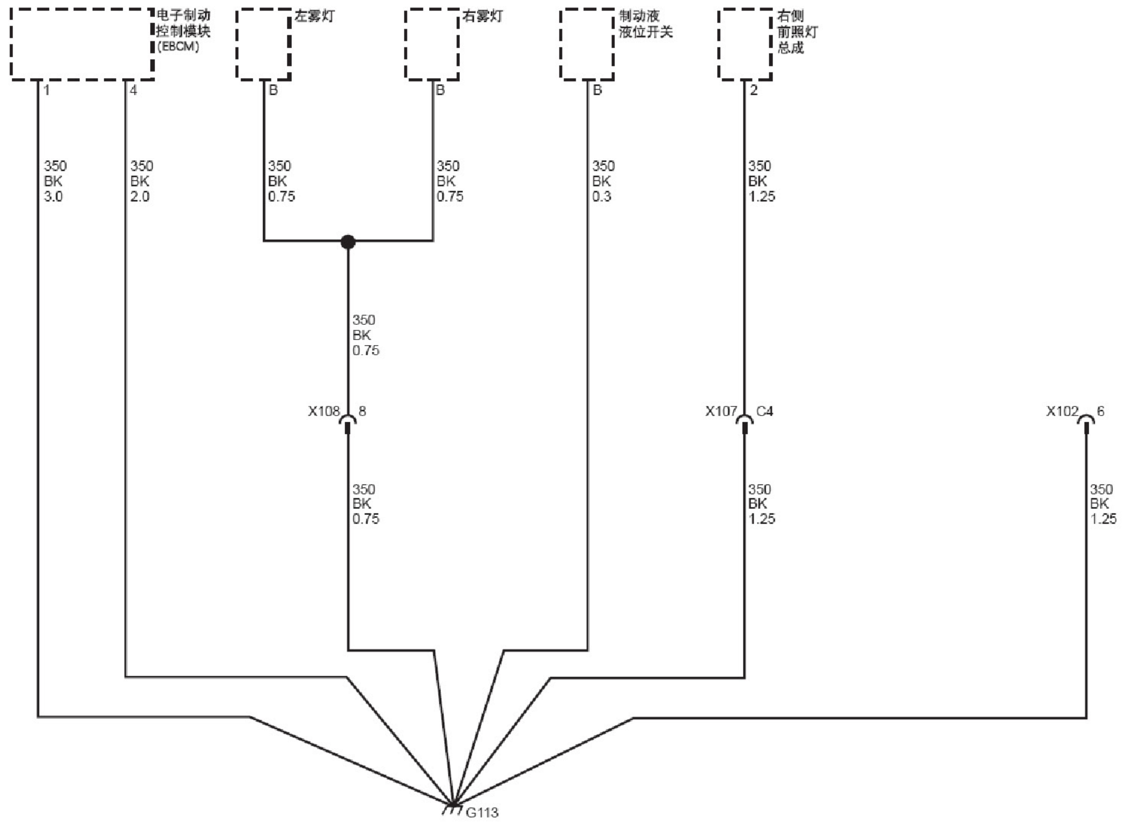
搭铁分布示意图 (G113)
