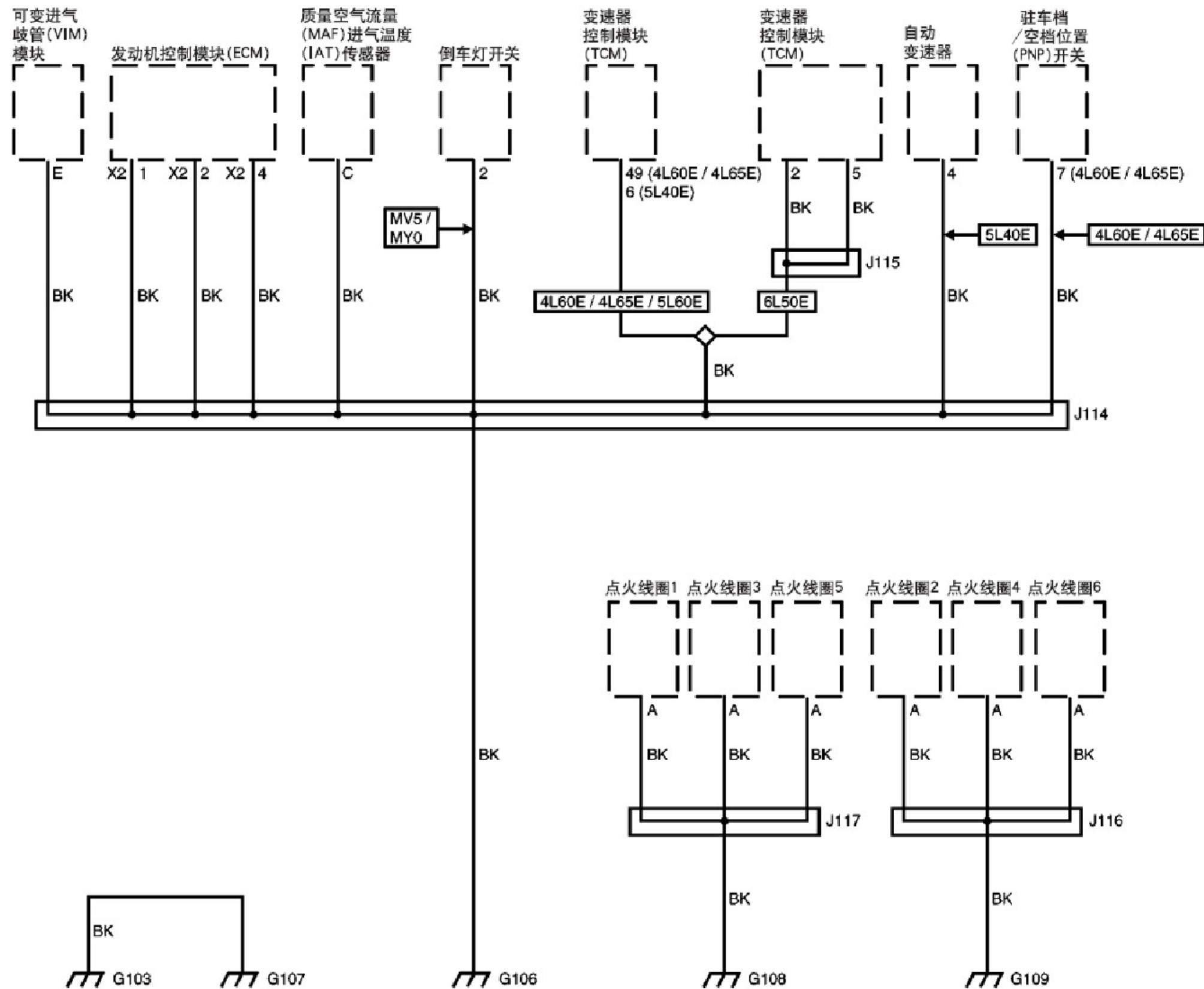
搭铁分布示意图 (G103、G106、G107、G108 和 G109 (LY7))
