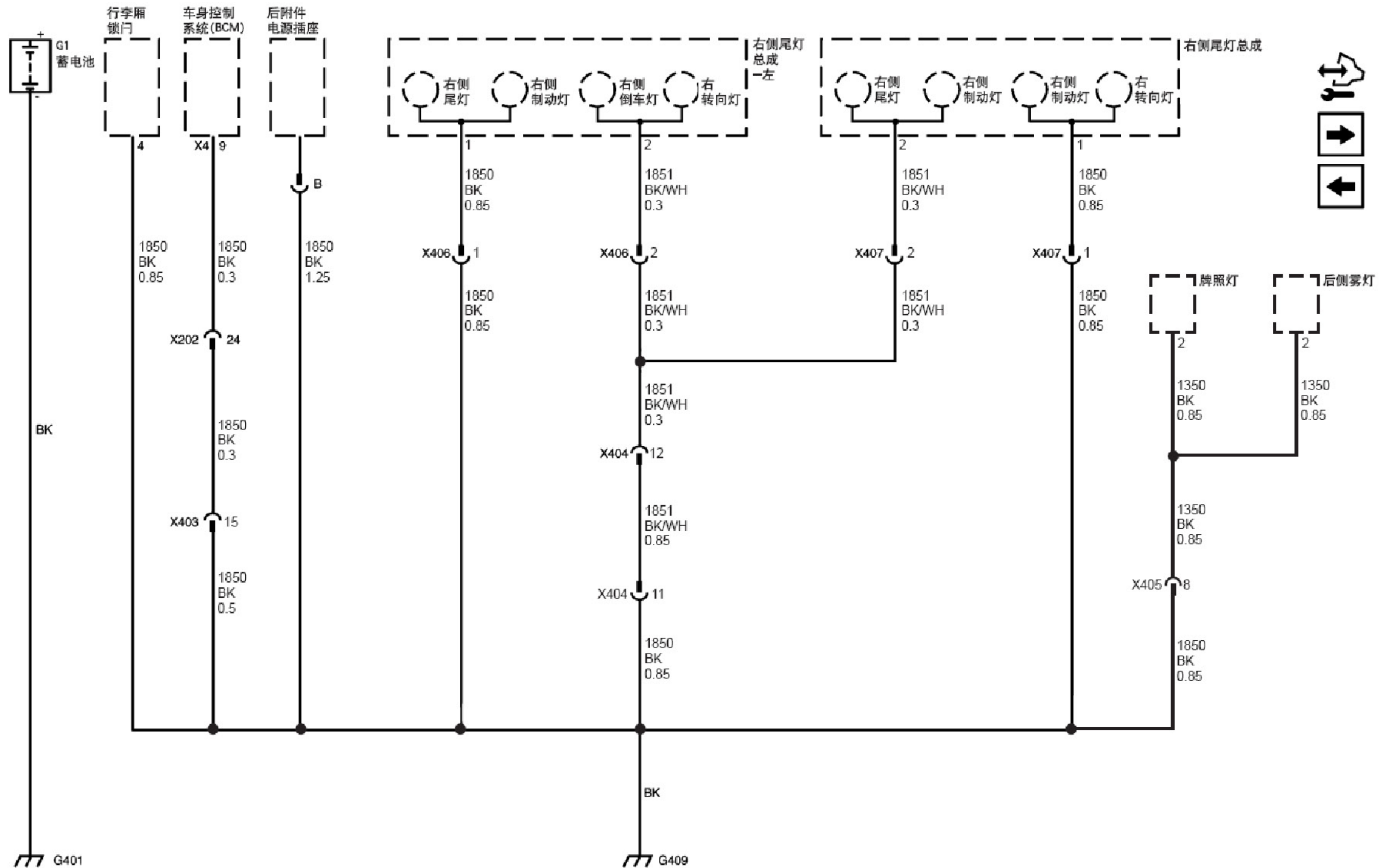
搭铁分布示意图 (G401 和 G409)
