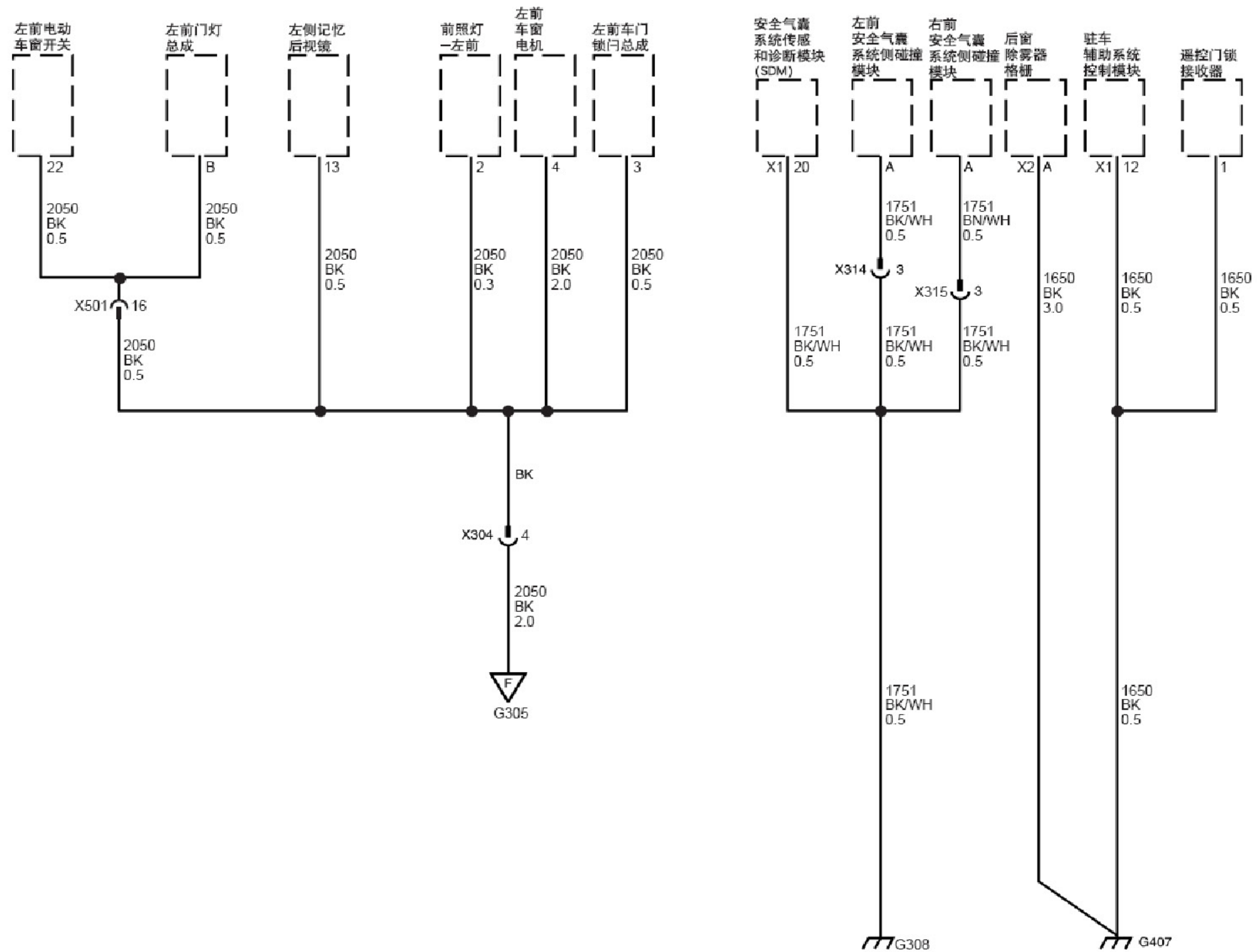
搭铁分布示意图 (G305 第 2 页, 共 2 页, G306 和 G407)
