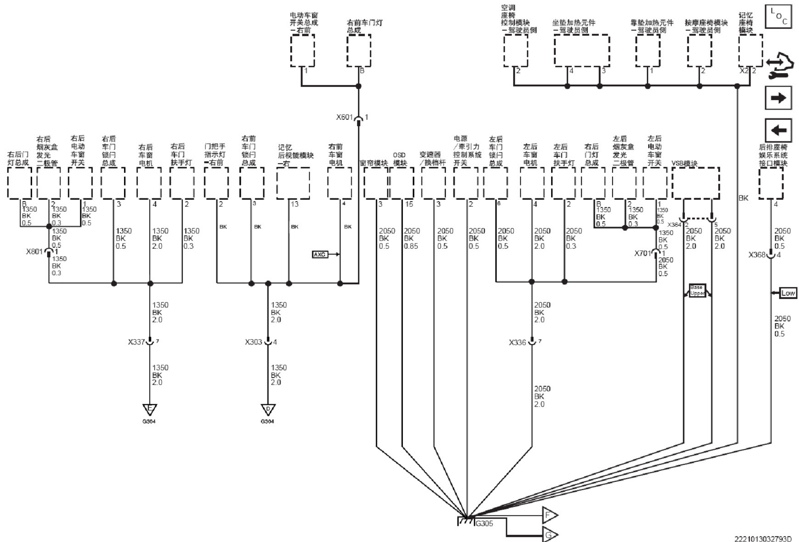
搭铁分布示意图 (G304 第 2 页, 共 2 页和 G305 第 1 页, 共 2 页)
