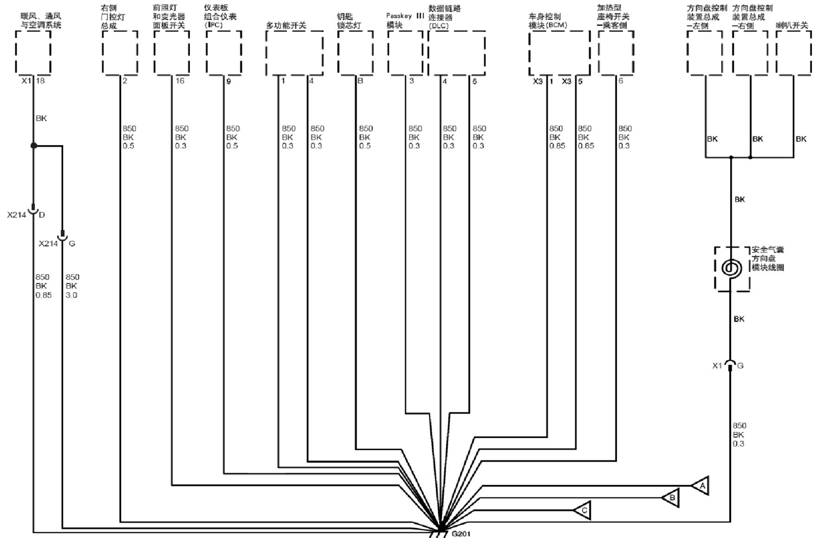
搭铁分布示意图 (G200、G201 第 1 页, 共 2 页)
