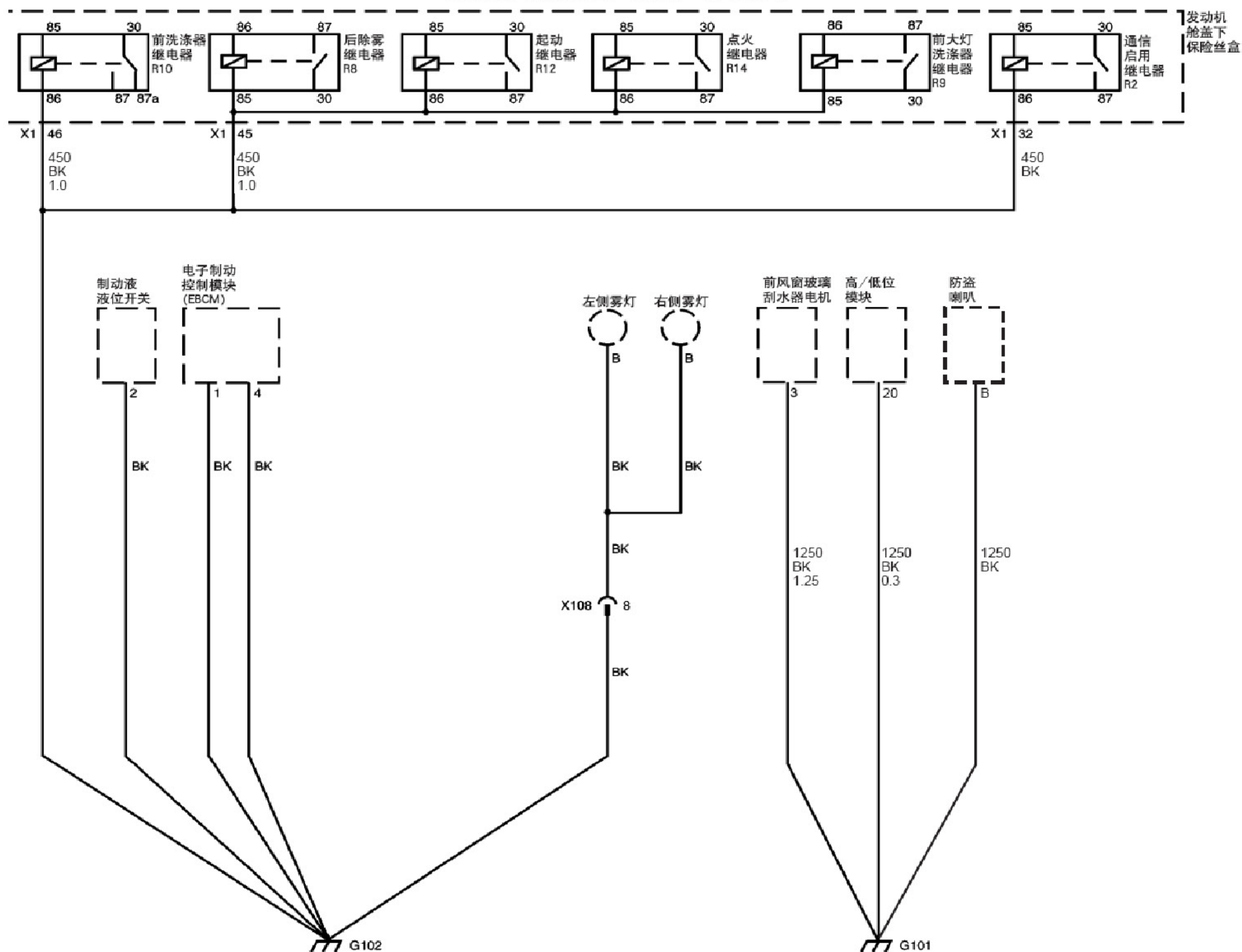
搭铁分布示意图 (G101 和 G102)
