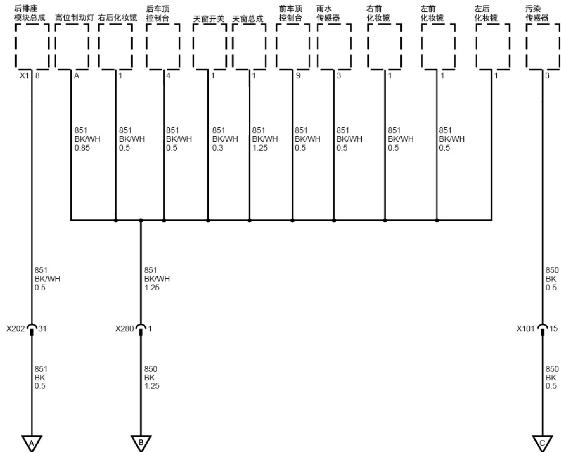
搭铁分布示意图 (G200、G201 第 2 页, 共 2 页)
