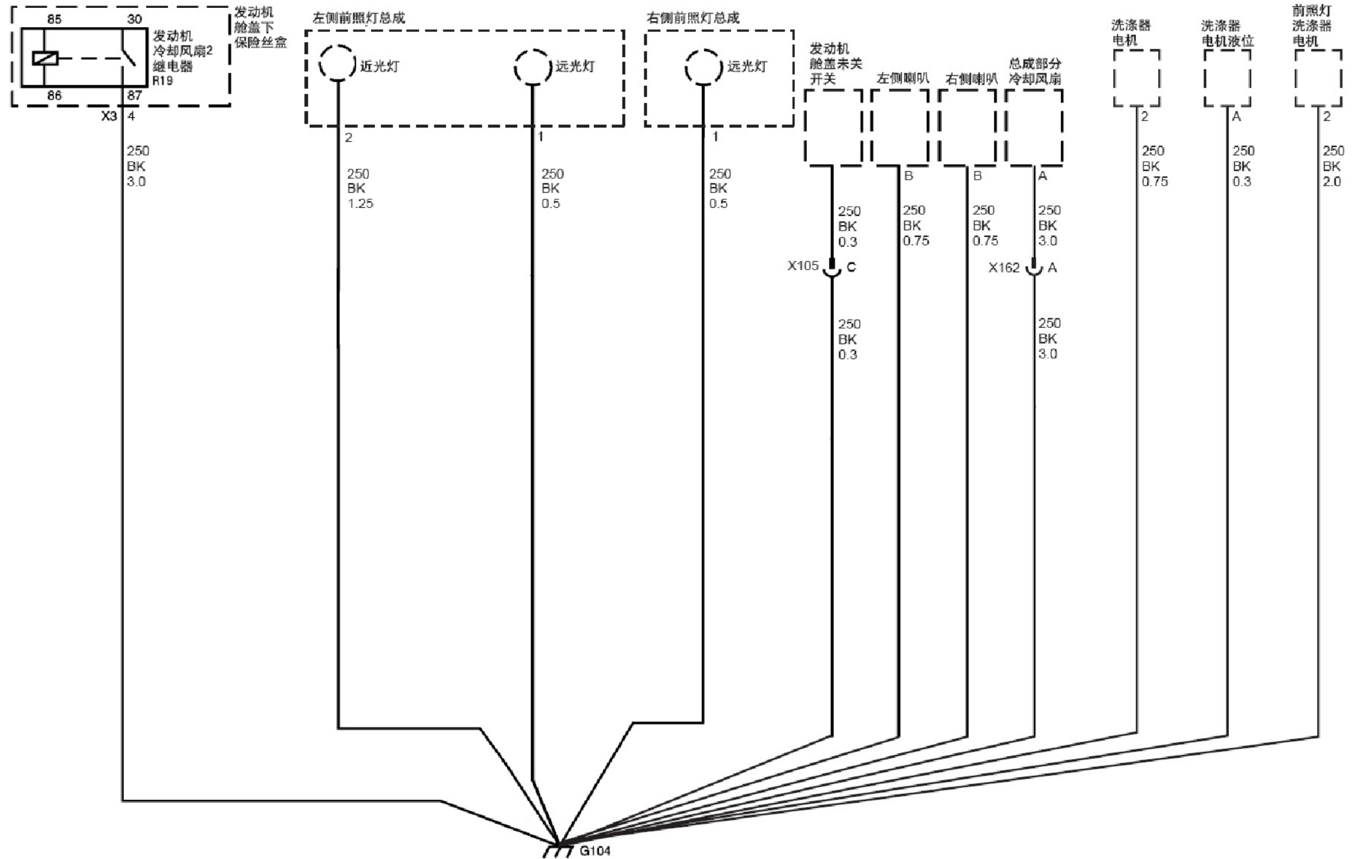
搭铁分布示意图 (G104)
