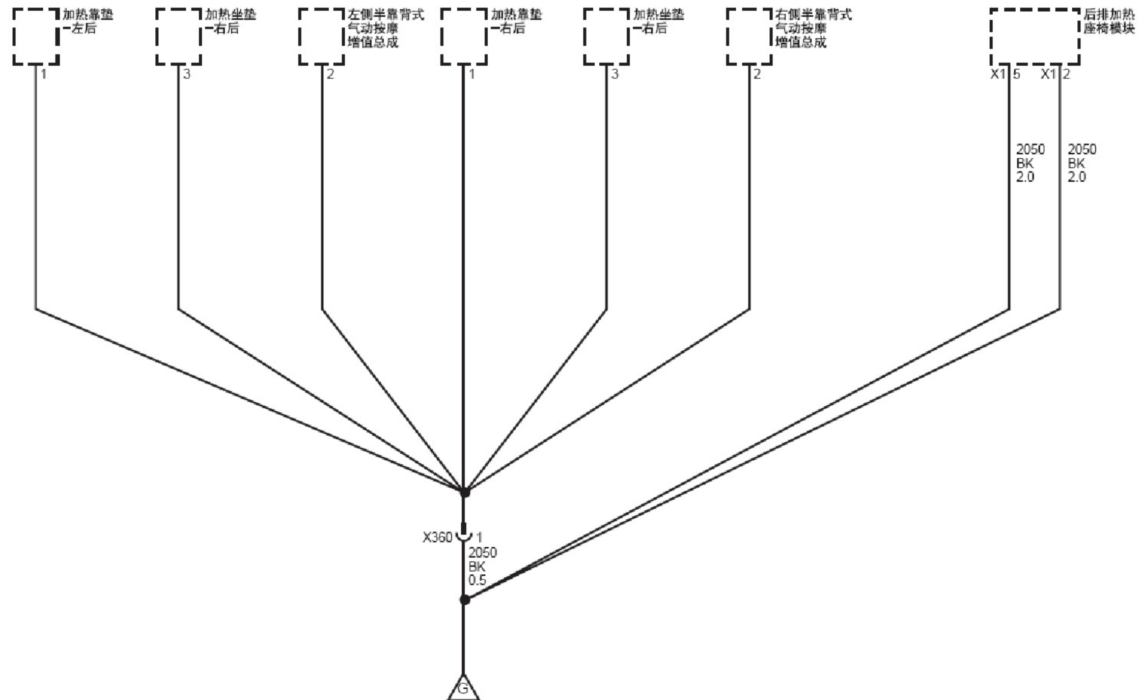
搭铁分布示意图 (G305 第 2 页, 共 2 页)
