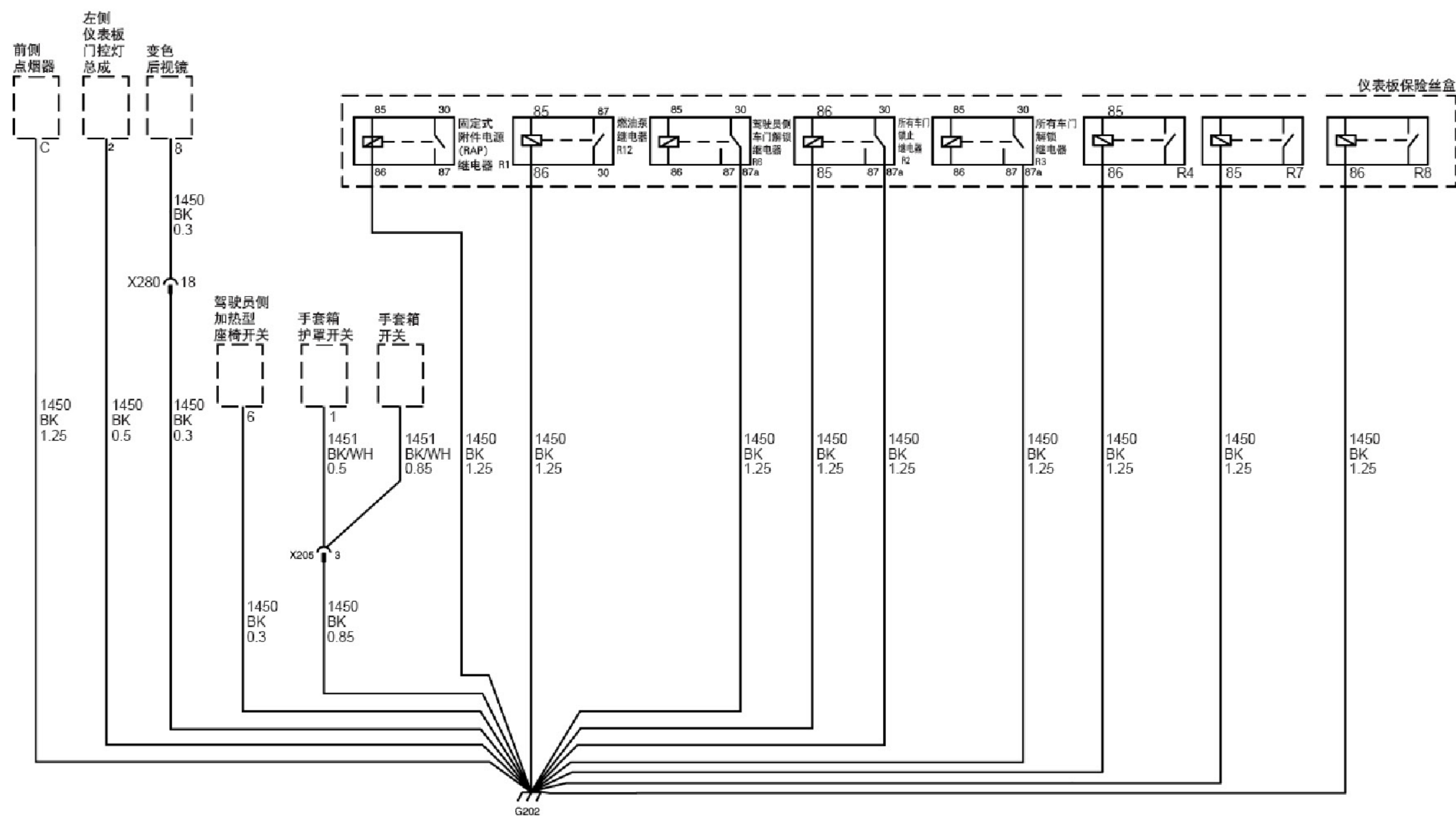
搭铁分布示意图 (G202)
