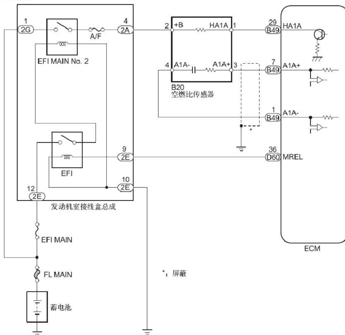
电路图
