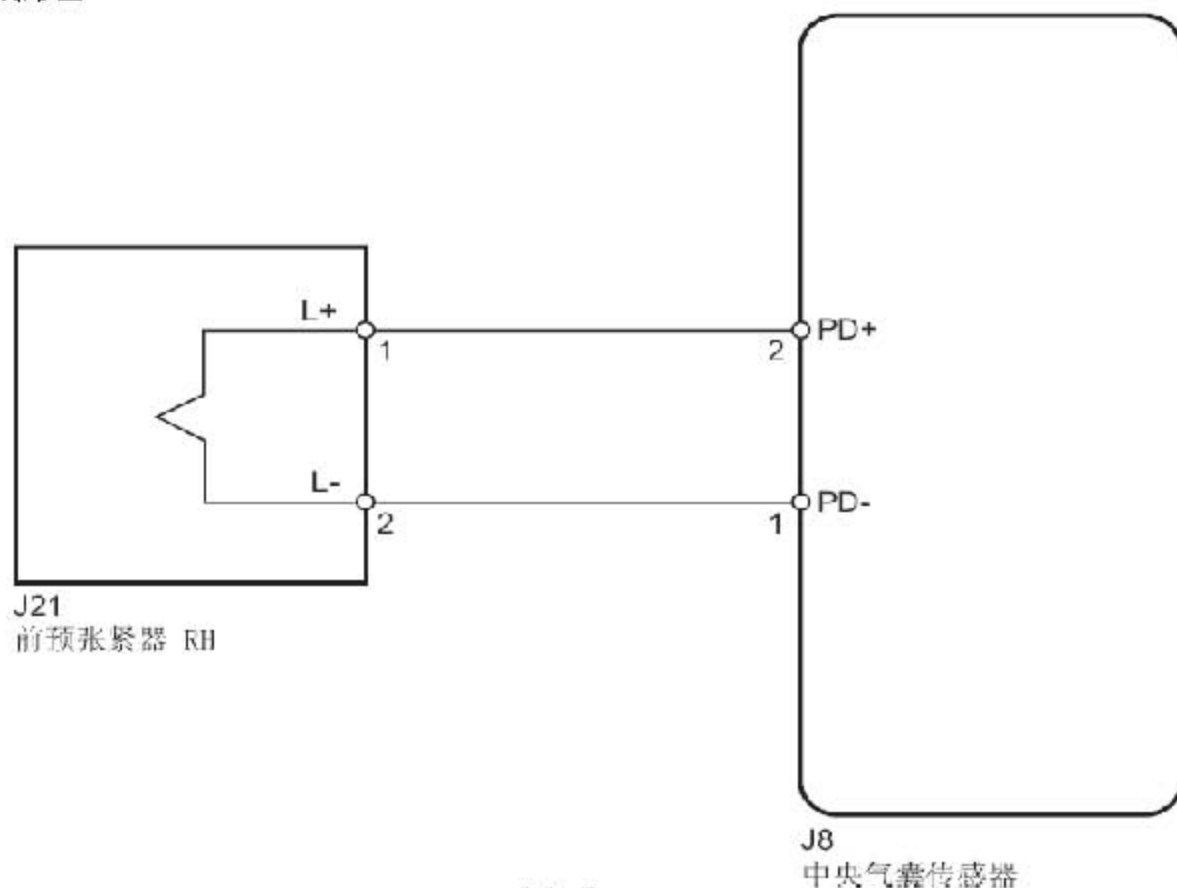
线路图
