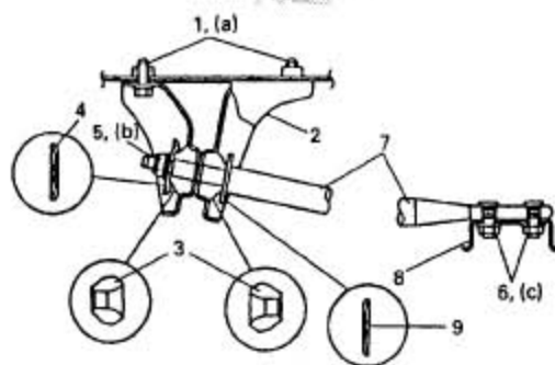
1. 压杆支架安装螺栓 2. 压杆支架 3. 压杆衬套 4. 压杆后垫圈 5. 压杆后螺母 6. 压杆前螺母 7. 压杆 8. 悬架摆臂 9. 压杆前垫圈
