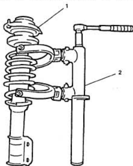
1. 前支柱总成 2. 弹簧压缩器
