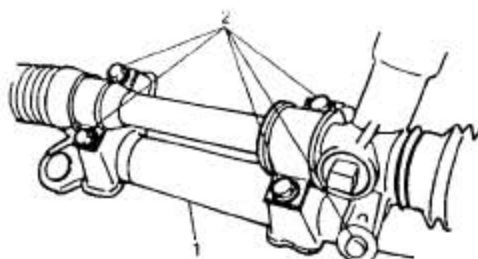
1. 悬架支架 2. 转向齿轮箱壳安装螺栓
