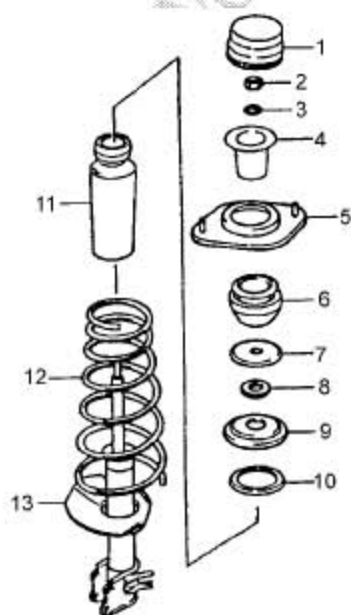
1. 支柱防尘罩 8. 支柱轴承 2. 支柱螺母 9. 弹簧上支座 3. 支柱锁紧垫圈 10. 支柱弹簧橡胶座 4. 减振器固定座 11. 防撞垫 5. 支柱支撑 12. 螺旋弹簧 6. 支柱内支撑 13. 前支柱总成 7. 支柱轴承座
